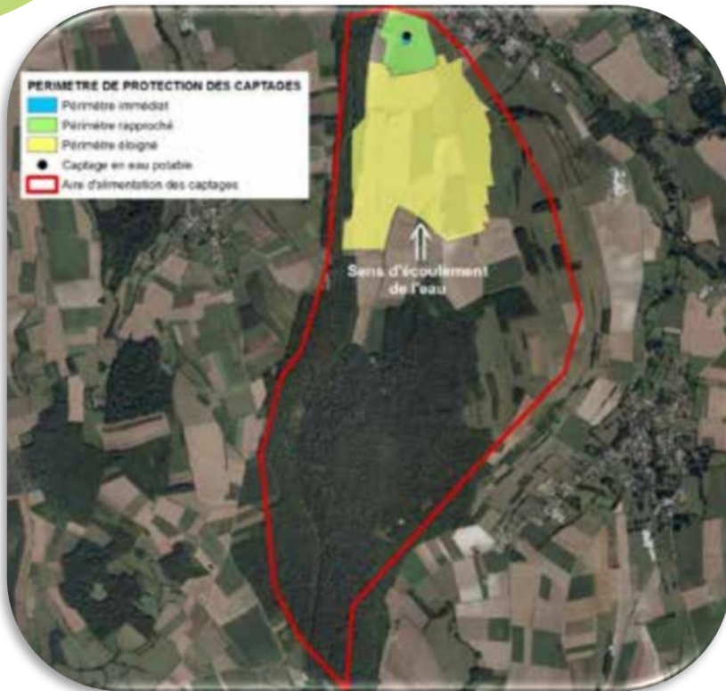
Protection des captages d'eau potable : délimitation des aires d'alimentation de captage / Périmètres de protection
